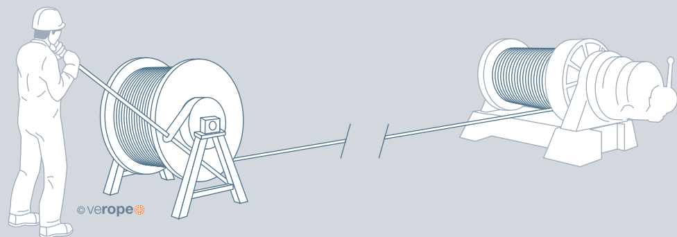
Fig. 31: Brake reels
