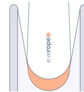
La luz es claramente visible entre la parte inferior de la galga y la ranura de la polea: la galga para ranura utilizada es demasiado grande.
